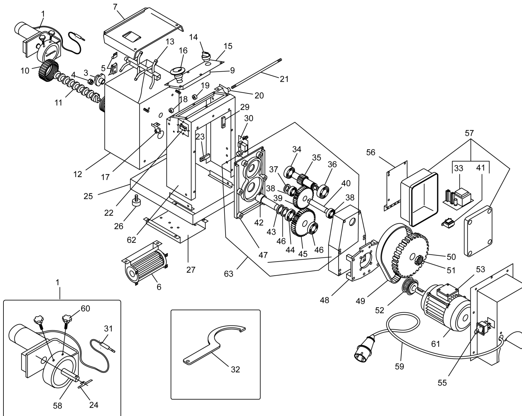
TAVOLA RICAMBI SPARE PARTS
